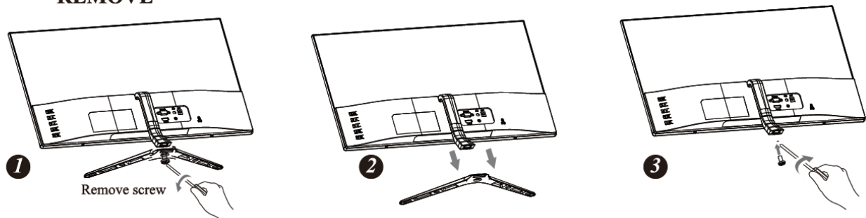
Figura 1. Instalar y desinstalar la base
